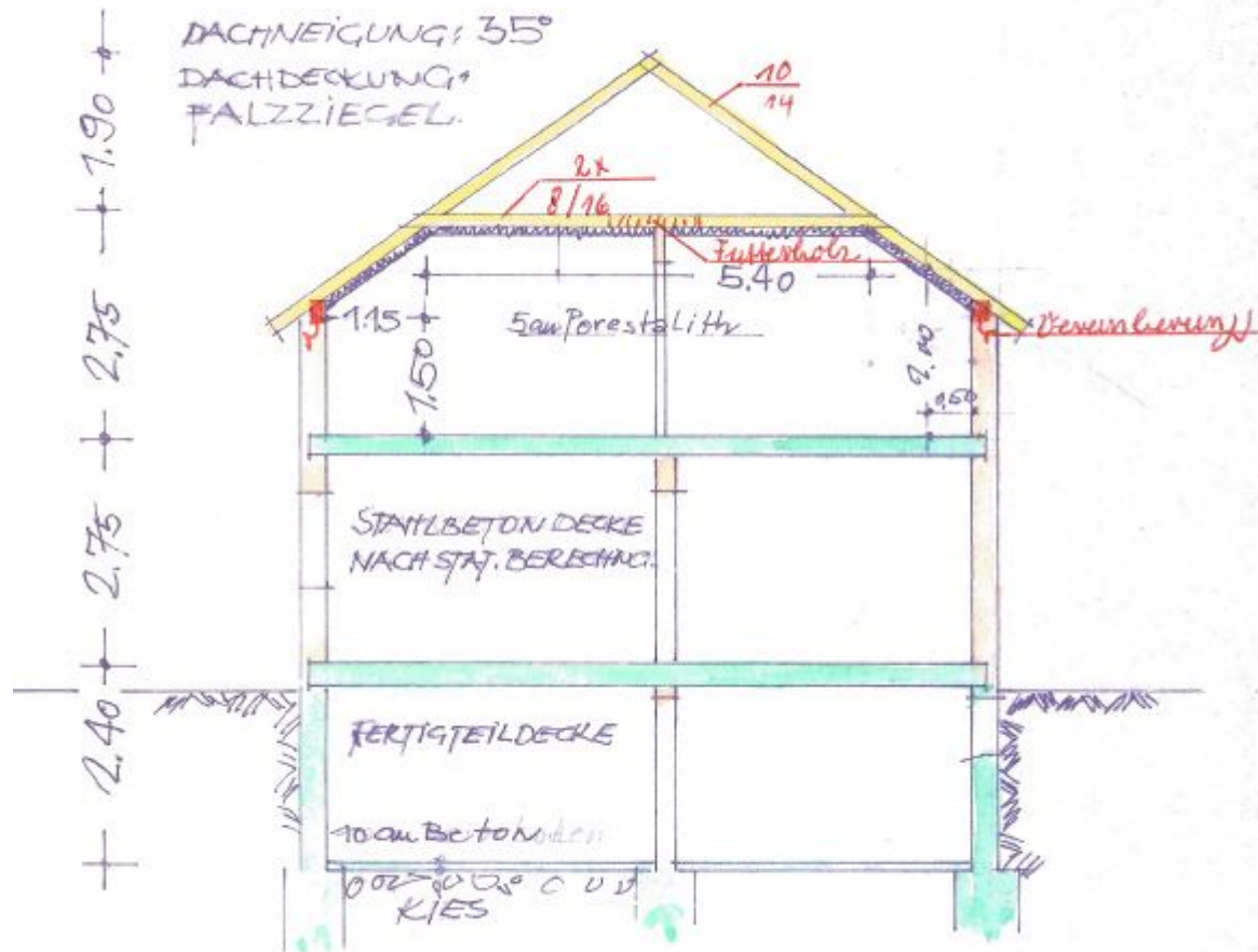
SCHNITT
